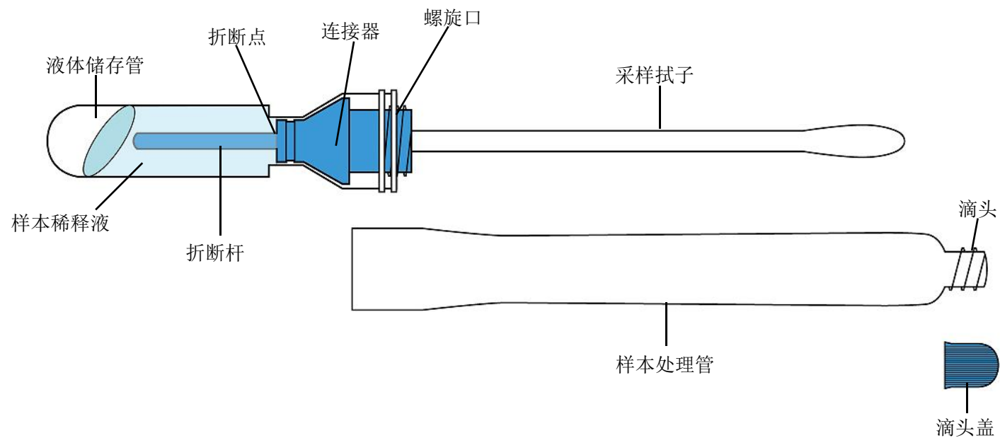
图 2: 采集器分解图
